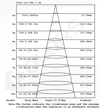
平均有效照度图
