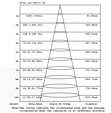
平均有效照度图
