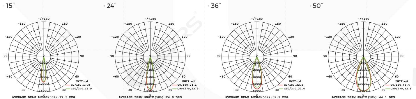
配光曲线
