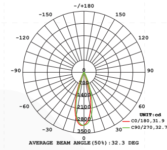
配光曲线
