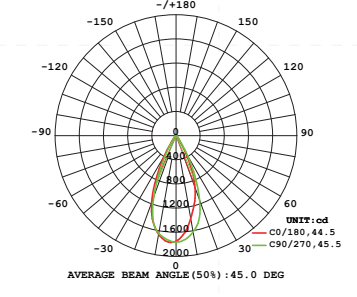
配光曲线
