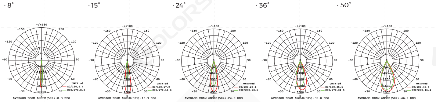
配光曲线
